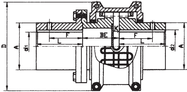
JS3501~JS3519 结构图
